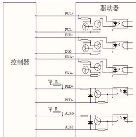
图 3 输入信号差分接法
