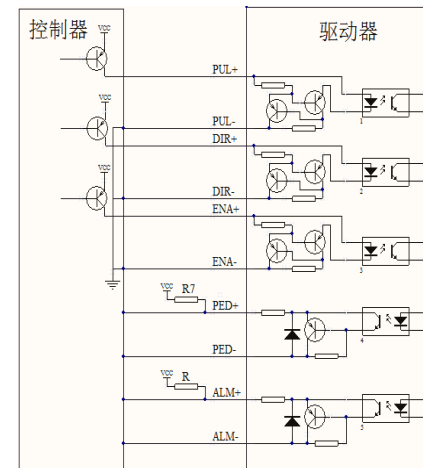
图 4 输入信号单端共阳极接法
