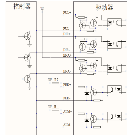
图 4 输入信号单端共阳极接法
