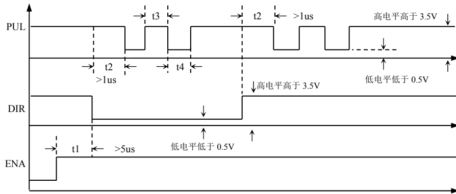
图 7 控制信号时序图
